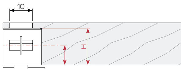
SENZA COLLARE WITHOUT COLLAR
