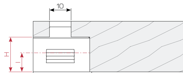
CON COLLARE CON CODOLO WITH COLLAR WITH DOWEL
