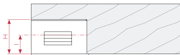
CON COLLARE SENZA CODOLO WITH COLLAR WITHOUT DOWEL
