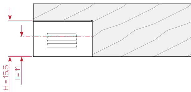
STANDARD SENZA CODOLO STANDARD WITHOUT DOWEL
