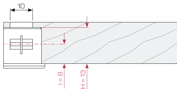
CON COLLARE WITH COLLAR
